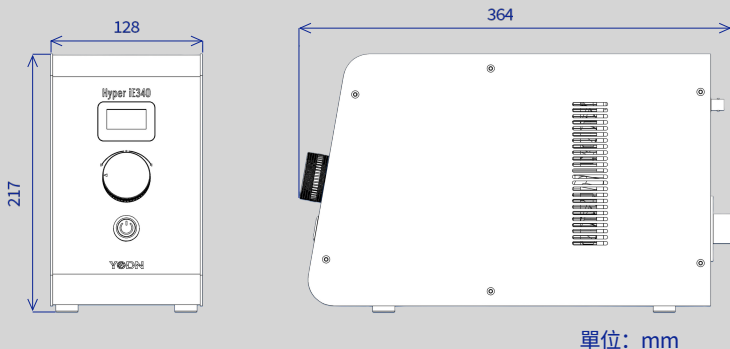
外觀尺寸
