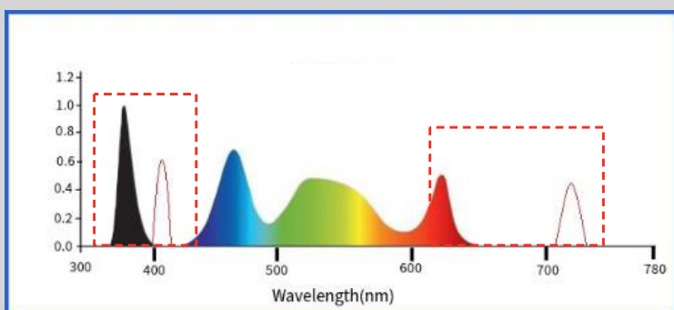
光譜圖
